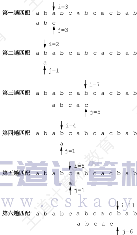
图 4.2 简单模式匹配算法举例
