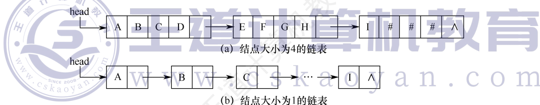
图 4.1 串值的链式存储方式
